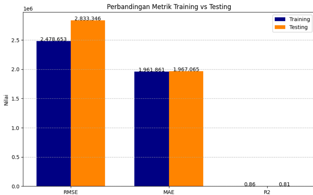
Gambar 4. 8 Perbandingan evaluasi testing dan training
