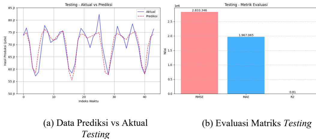
Gambar 4. 7 Grafik Hasil Evaluasi Testing Model
