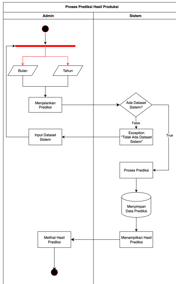
Gambar 3. 6 Activity Proses Prediksi Hasil Produksi
