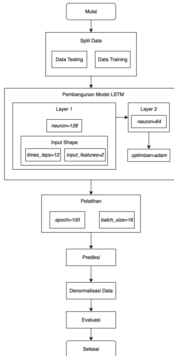
Gambar 3. 3 Desain Model Prediksi
