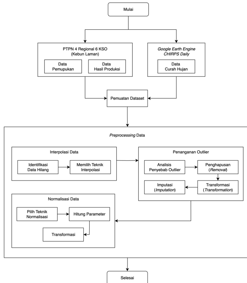
Gambar 3. 2 Desain Pengelolaan Data
